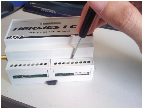
Retirar la tapa de las bornas.
